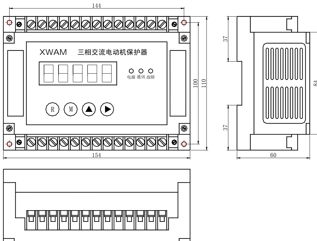
AMDG-X/E41□ 系列电动机保护器主单元外形及安装孔尺寸
