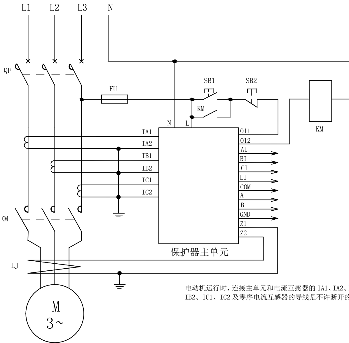
AMDG-X/E41□ 系列电动机保护器应用电气原理图
