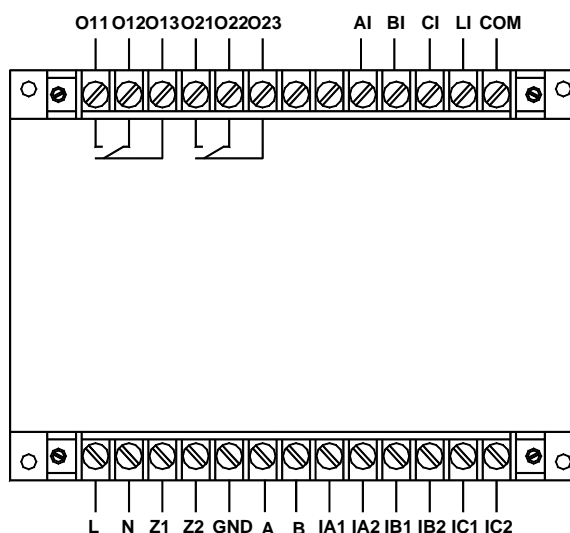
AMDG-X/E412 系列保护器主单元接线端子图
