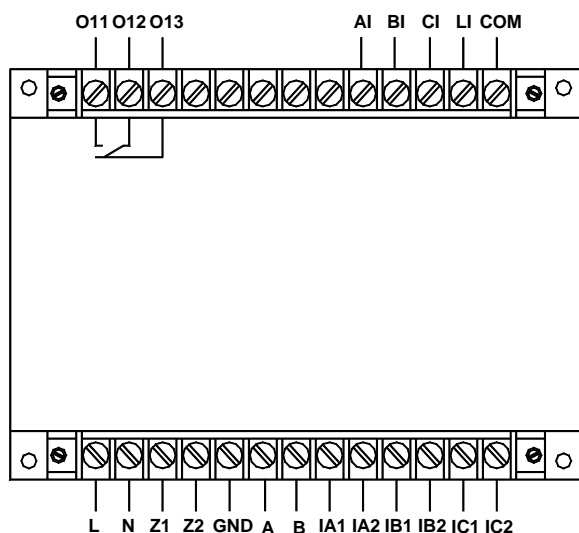
AMDG-X/E411 系列保护器主单元接线端子图
