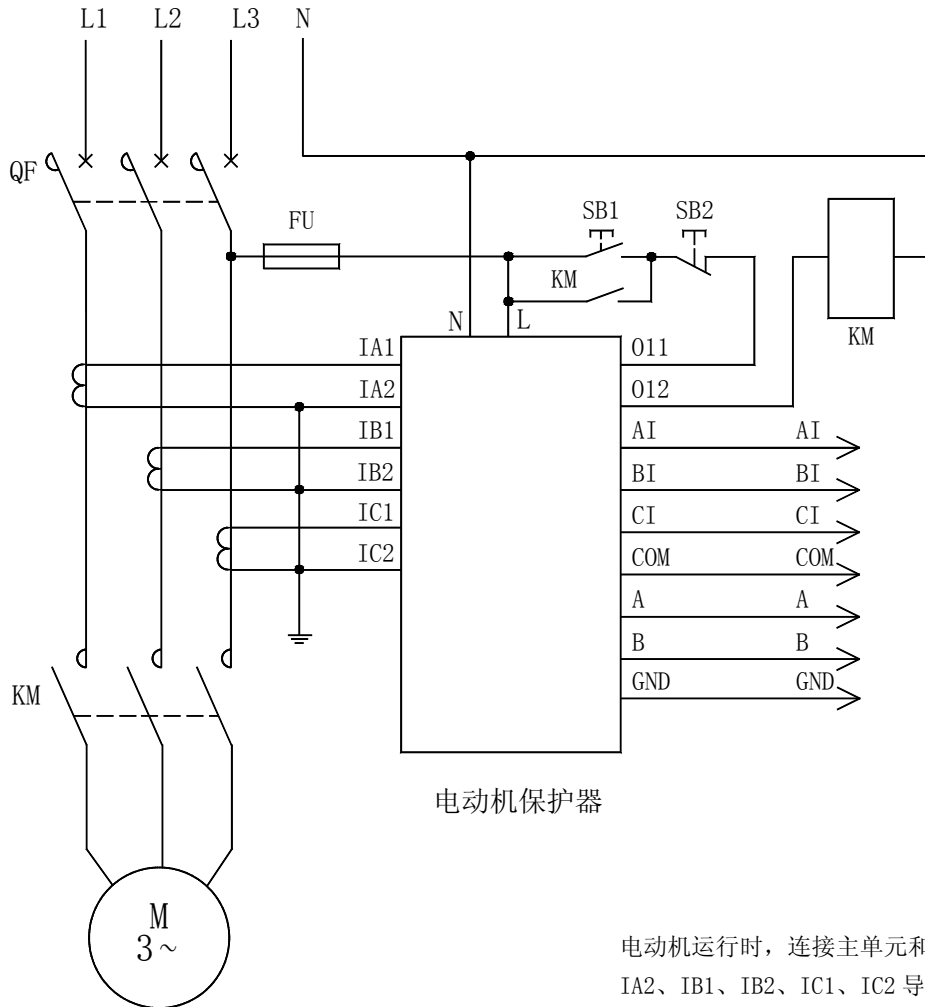
AMDG-X/E40□ 系列电动机保护器应用电气原理图
