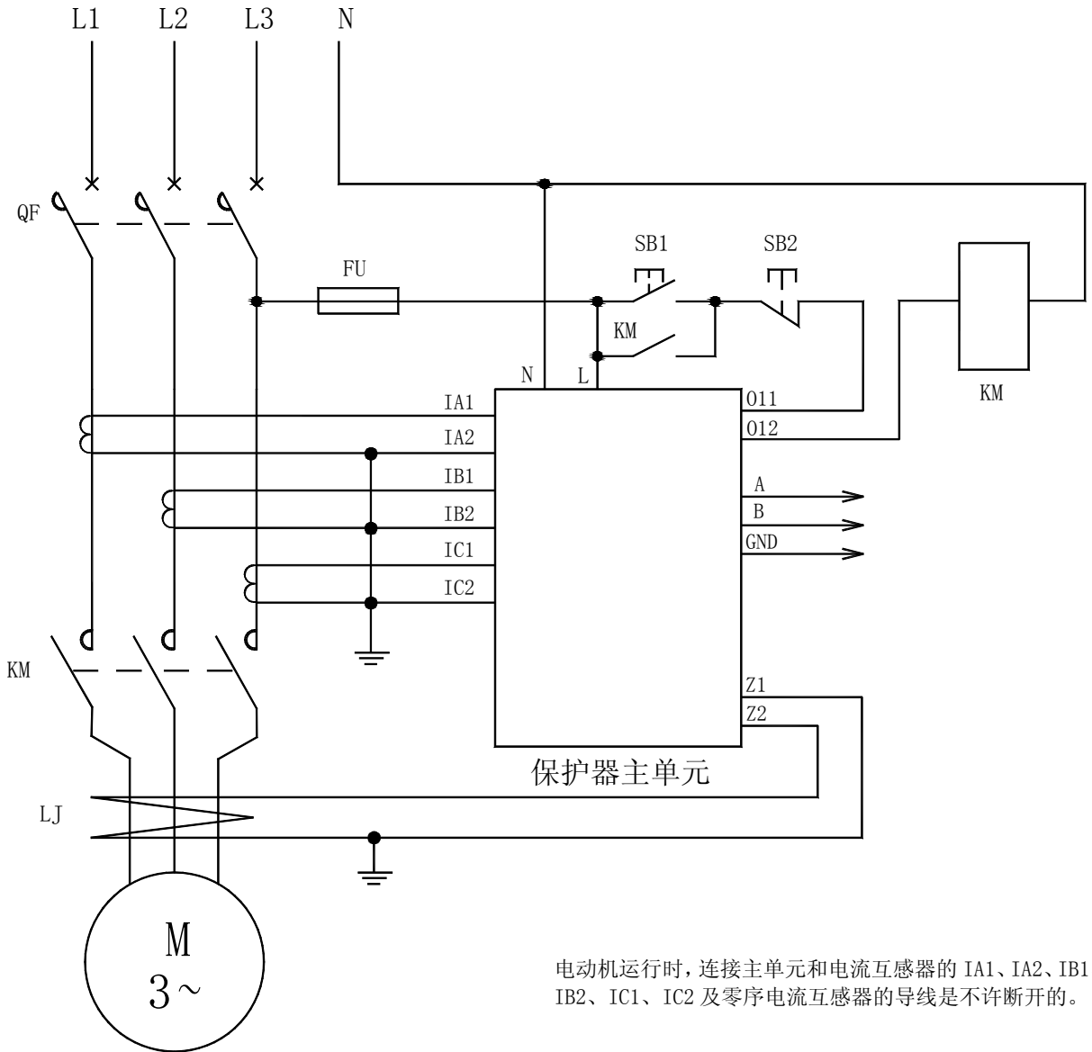
AMDG-X/E35□ 系列电动机保护器应用电气原理图
