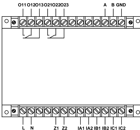
AMDG-X/E352 系列保护器主单元接线端子图
