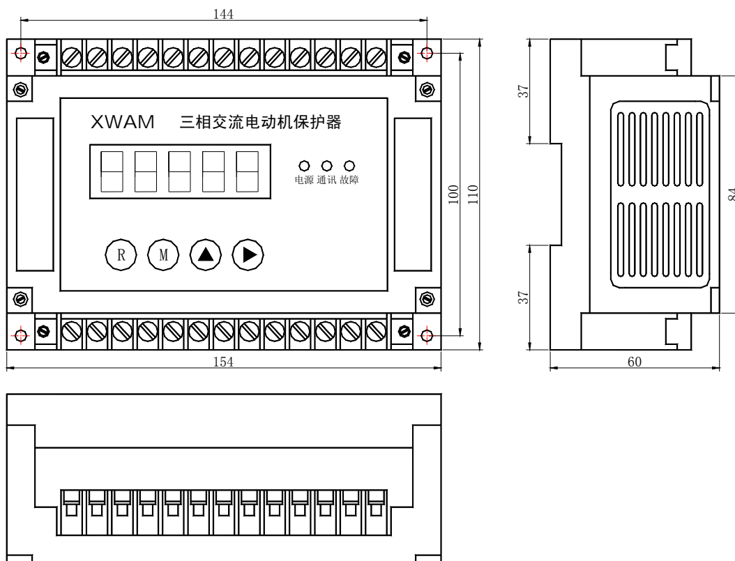
AMDG-X/E35□ 系列电动机保护器主单元外形及安装孔尺寸
