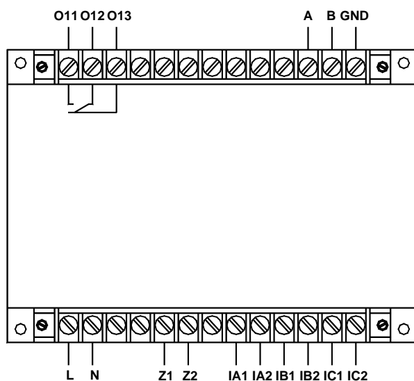
AMDG-X/E351 系列保护器主单元接线端子图
