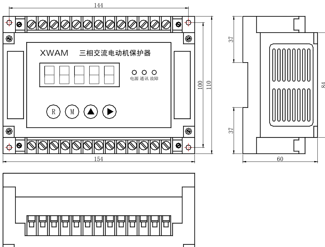
AMDG-X/E31□ 系列电动机保护器主单元外形及安装孔尺寸
