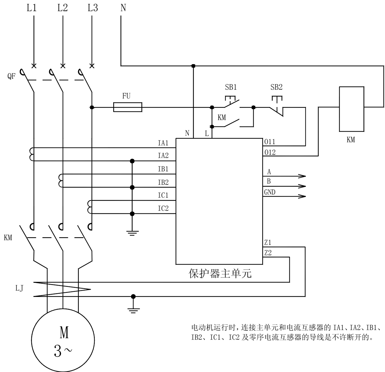
AMDG-X/E31□ 系列电动机保护器应用电气原理图
