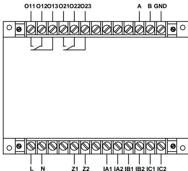
AMDG-X/E312 系列保护器主单元接线端子图
