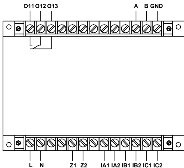
AMDG-X/E311 系列保护器主单元接线端子图
