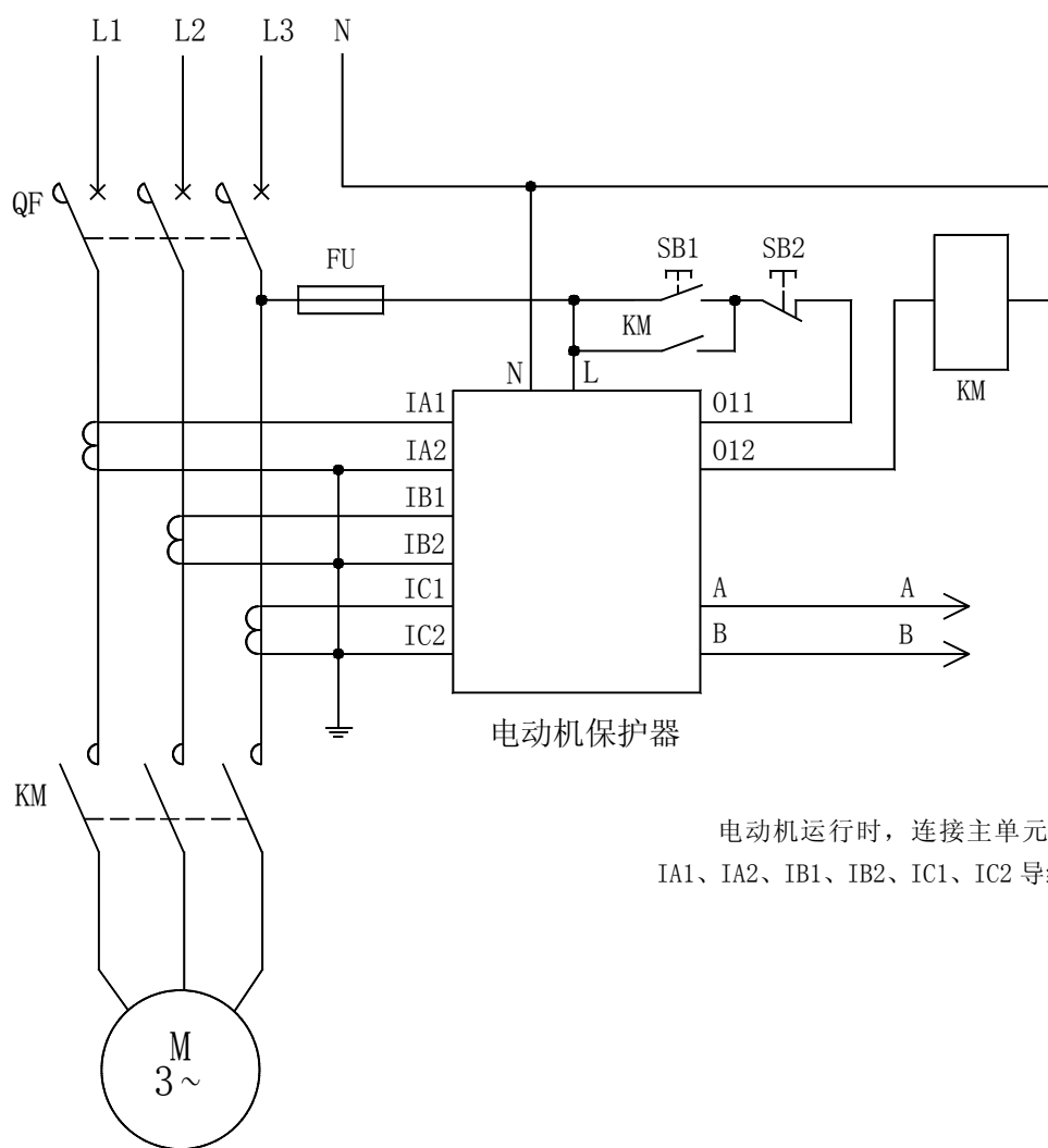
AMDG-X/E22□ 系列电动机保护器应用电气原理图
