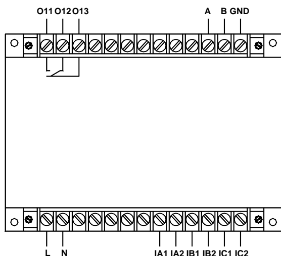
AMDG-X/E221 系列保护器主单元接线端子图
