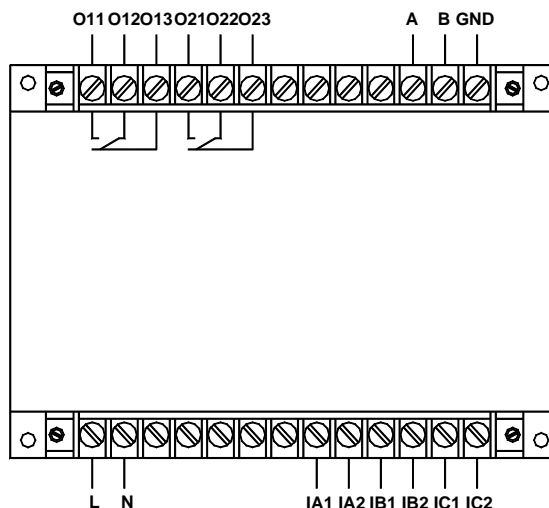
AMDG-X/E222 系列保护器主单元接线端子图
