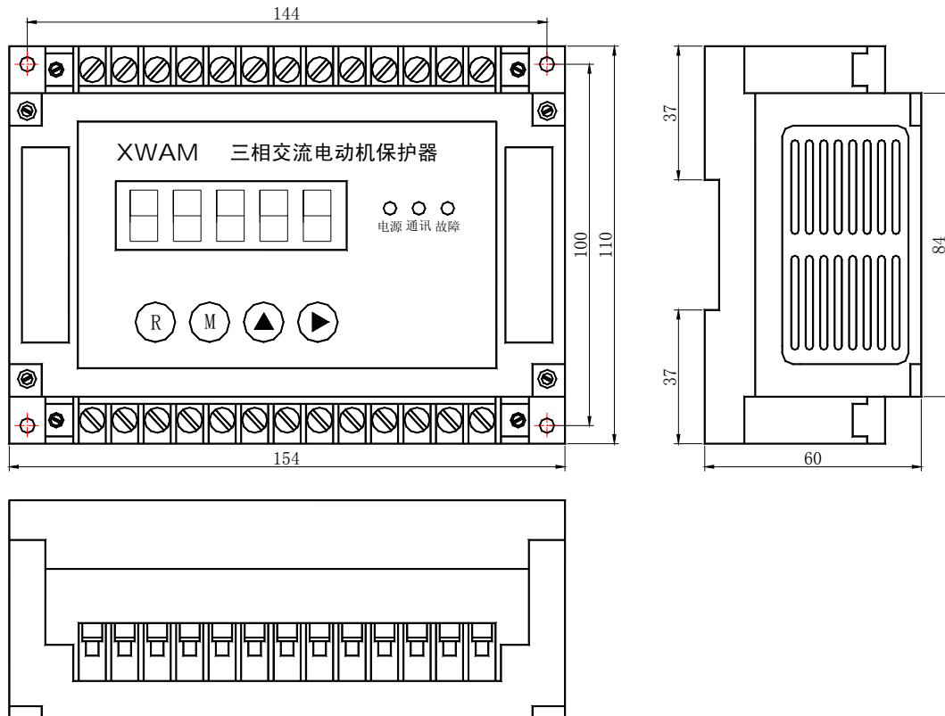
AMDG-X/E22□ 系列电动机保护器主单元外形及安装孔尺寸
