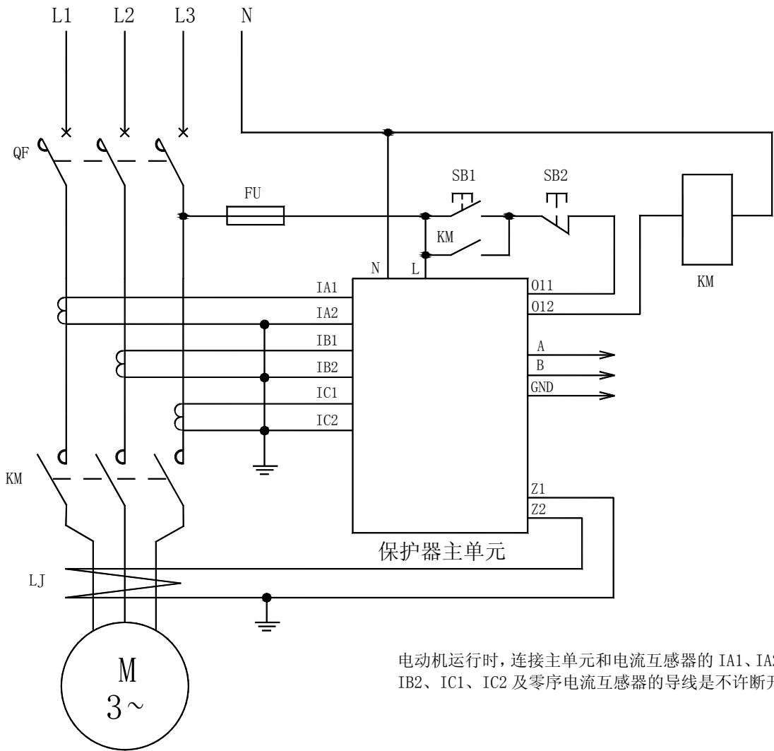
AMDG-X/E21□ 系列电动机保护器应用电气原理图
