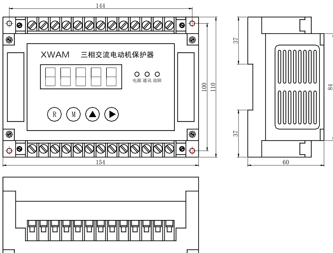
AMDG-X/E21□ 系列电动机保护器主单元外形及安装孔尺寸
