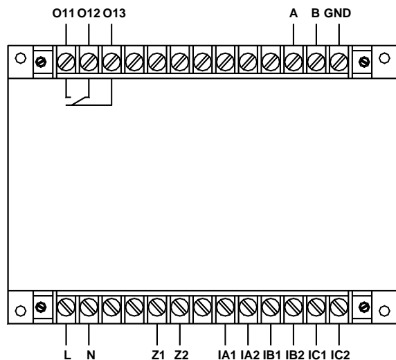
AMDG-X/E211 系列保护器主单元接线端子图
