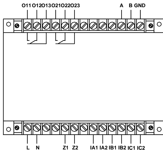
AMDG-X/E212 系列保护器主单元接线端子图
