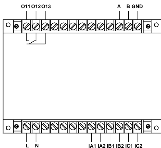
AMDG-X/E201 系列保护器主单元接线端子图
