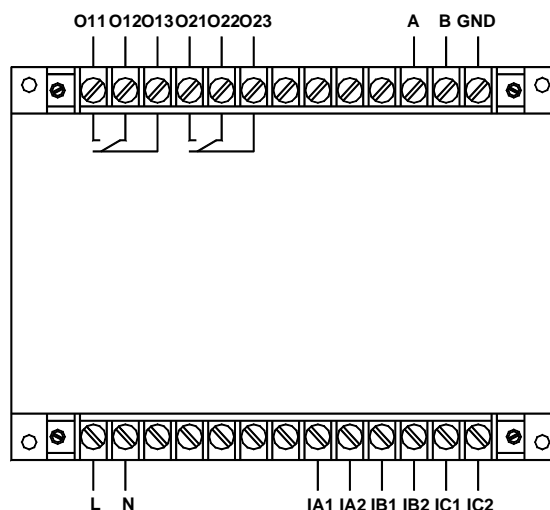
AMDG-X/E202 系列保护器主单元接线端子图
