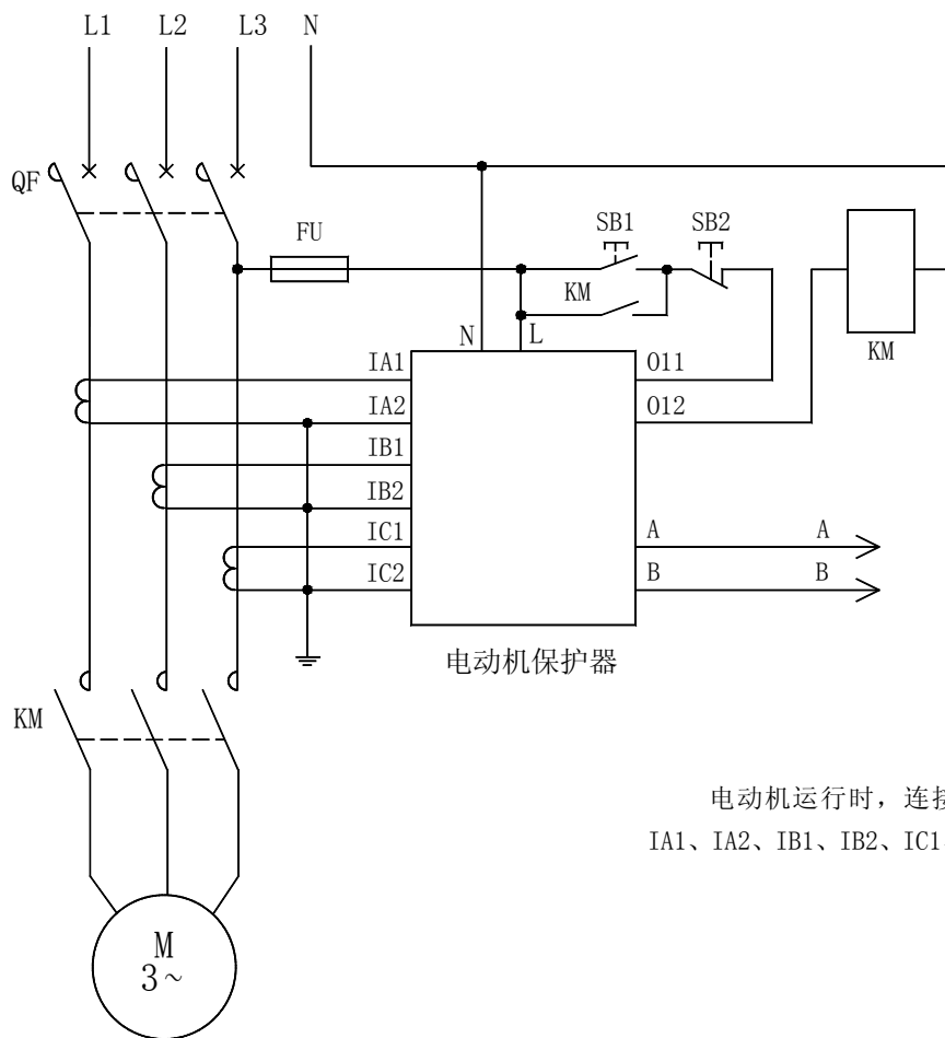
AMDG-X/E20□ 系列电动机保护器应用电气原理图
