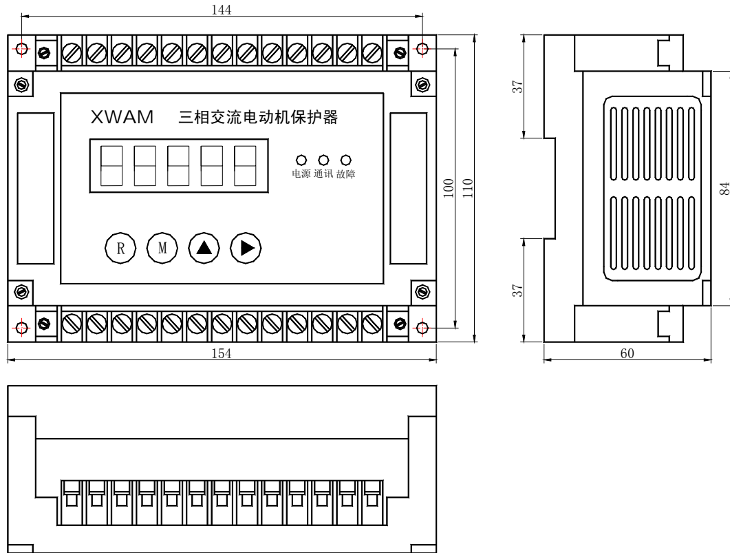
AMDG-X/E20□ 系列电动机保护器主单元外形及安装孔尺寸
