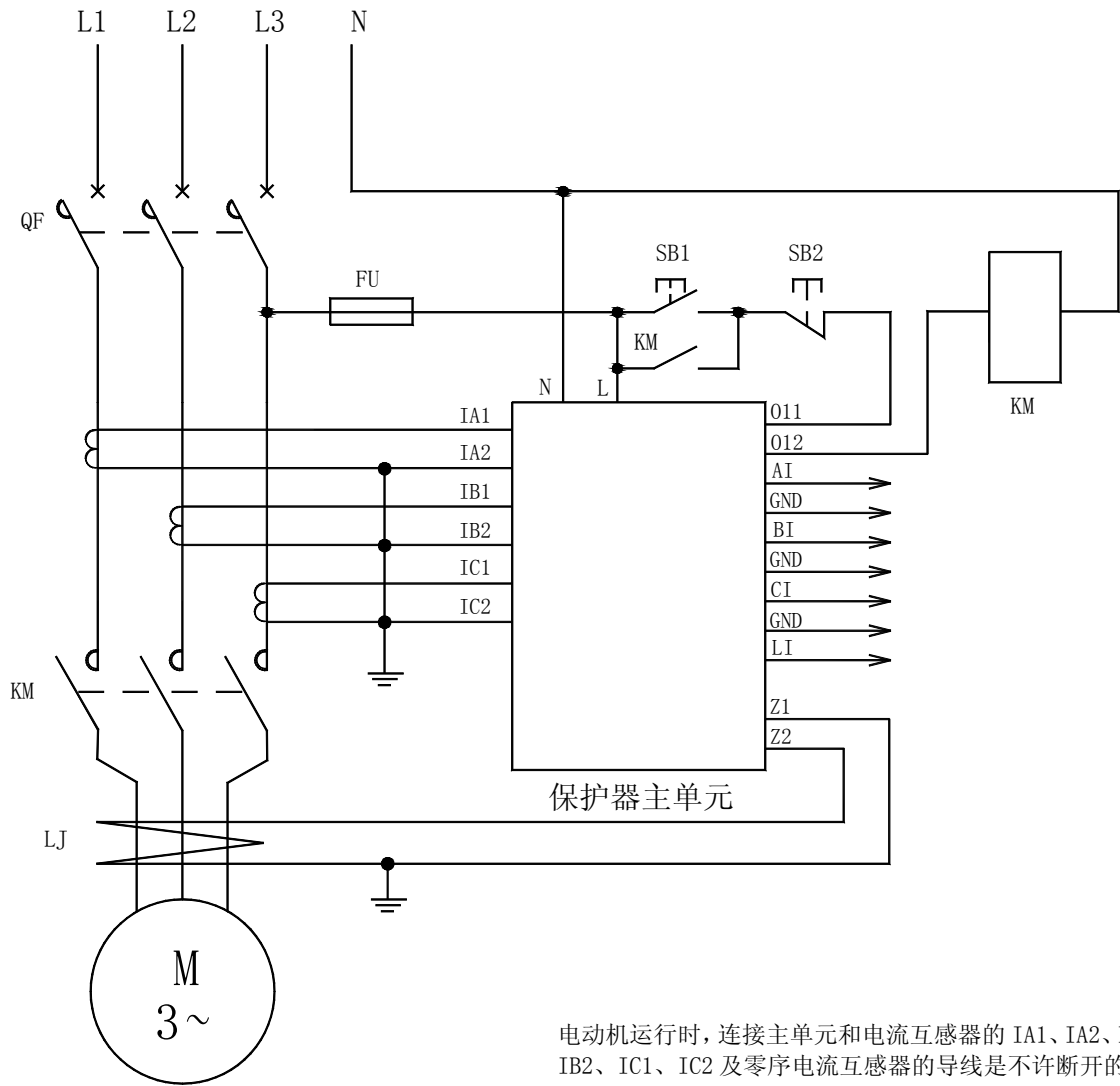
AMDG-X/E15□ 系列电动机保护器应用电气原理图
