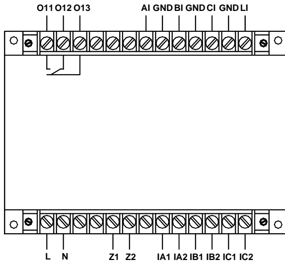
AMDG-X/E151 系列保护器主单元接线端子图
