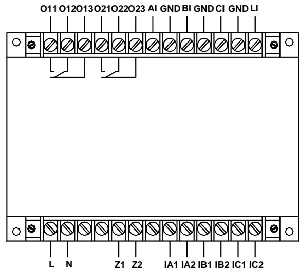
AMDG-X/E152 系列保护器主单元接线端子图
