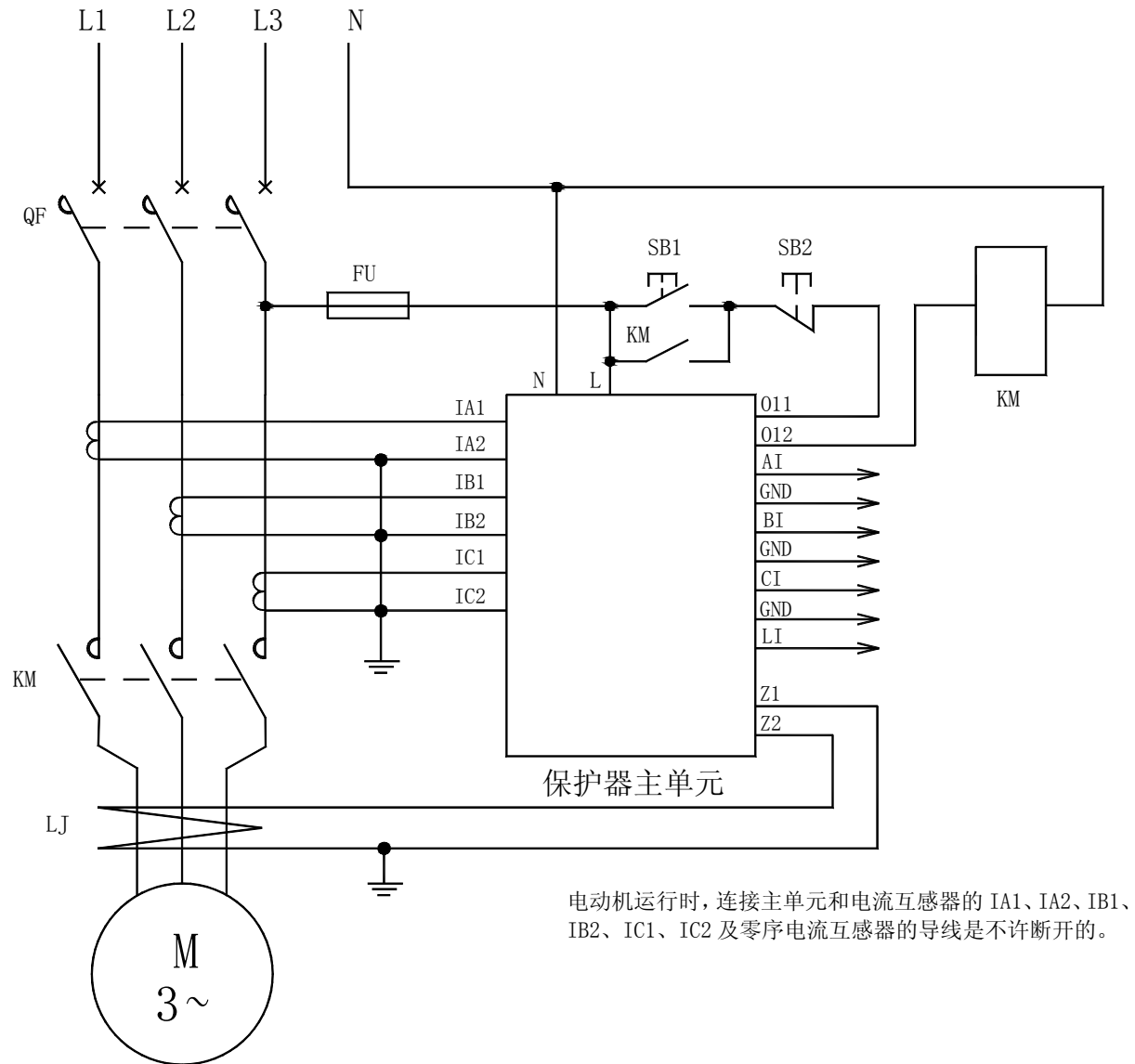
AMDG-X/E11□ 系列电动机保护器应用电气原理图
