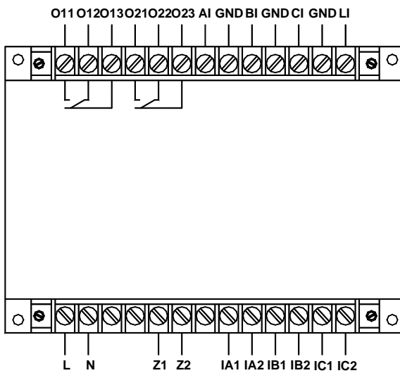
AMDG-X/E112 系列保护器主单元接线端子图
