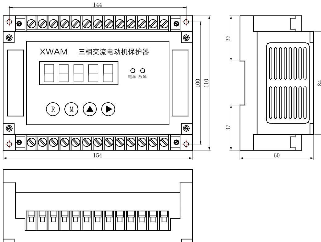
AMDG-X/E11□ 系列电动机保护器主单元外形及安装孔尺寸
