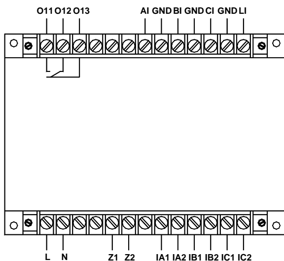
AMDG-X/E111 系列保护器主单元接线端子图
