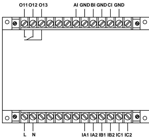
AMDG-X/E101 系列保护器主单元接线端子图
