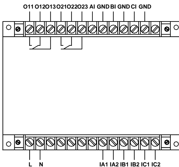
AMDG-X/E102 系列保护器主单元接线端子图
