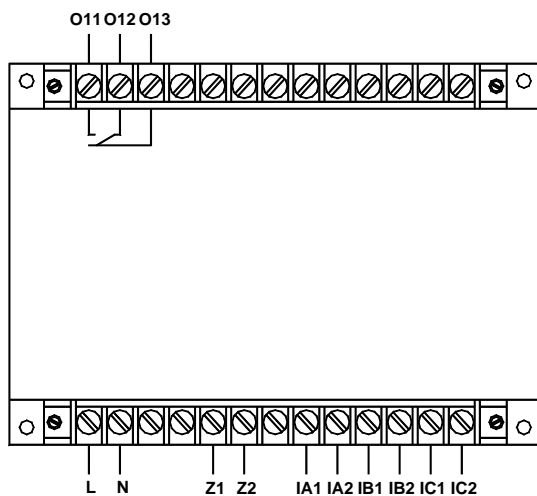
AMDG-X/E051 系列保护器主单元接线端子图
