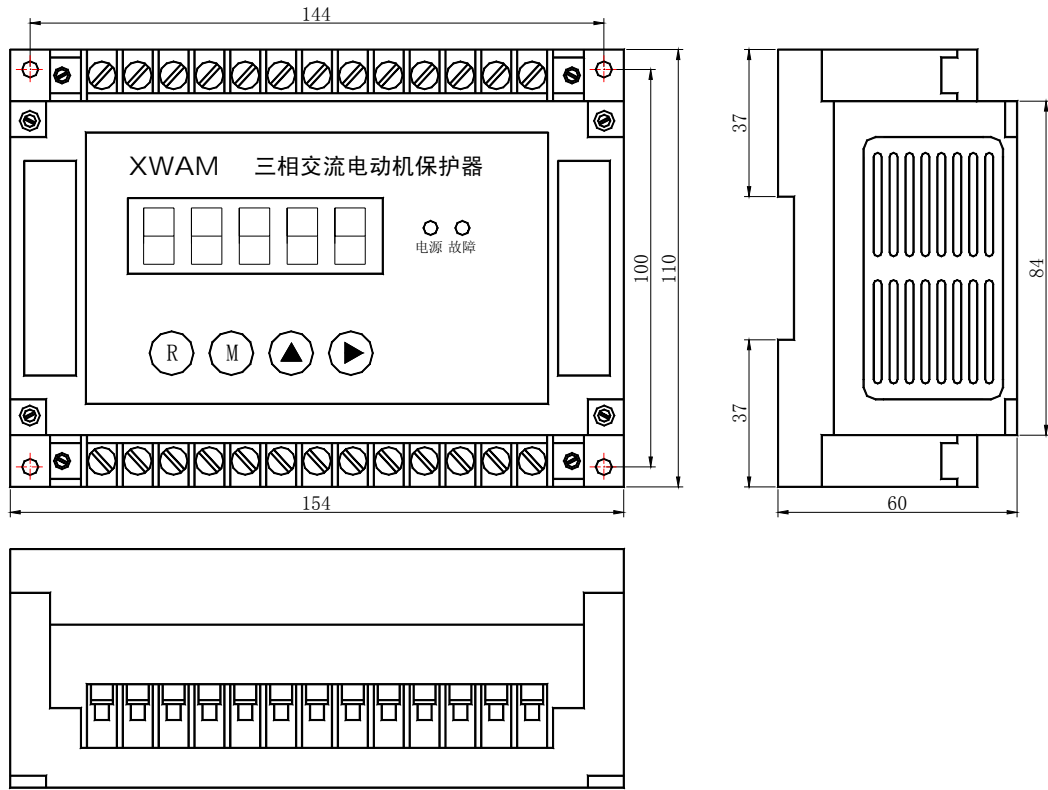
AMDG-X/E05□ 系列电动机保护器主单元外形及安装孔尺寸
