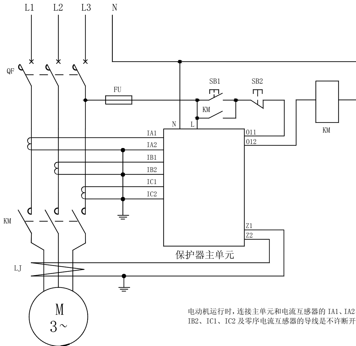
AMDG-X/E05□ 系列电动机保护器应用电气原理图
