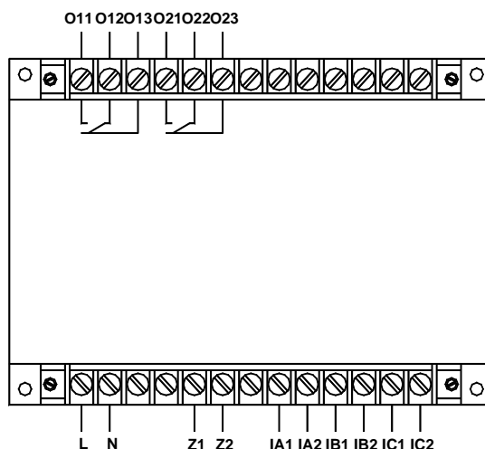
AMDG-X/E052 系列保护器主单元接线端子图
