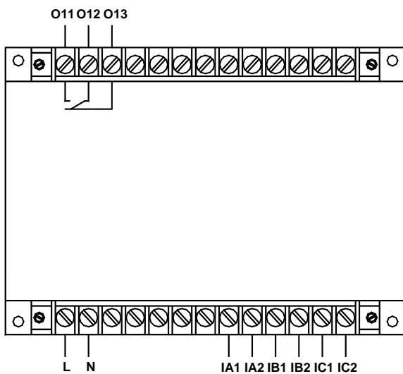
AMDG-X/E021 系列保护器主单元接线端子图
