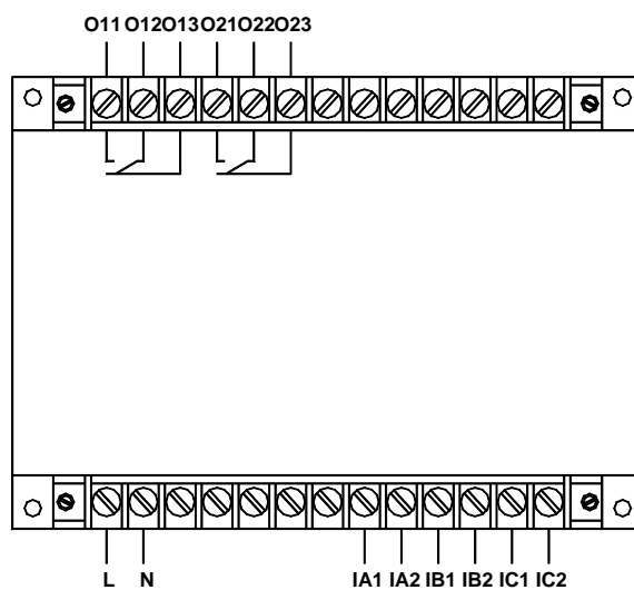
AMDG-X/E022 系列保护器主单元接线端子图
