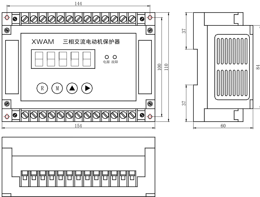
AMDG-X/E02□ 系列电动机保护器主单元外形及安装孔尺寸
