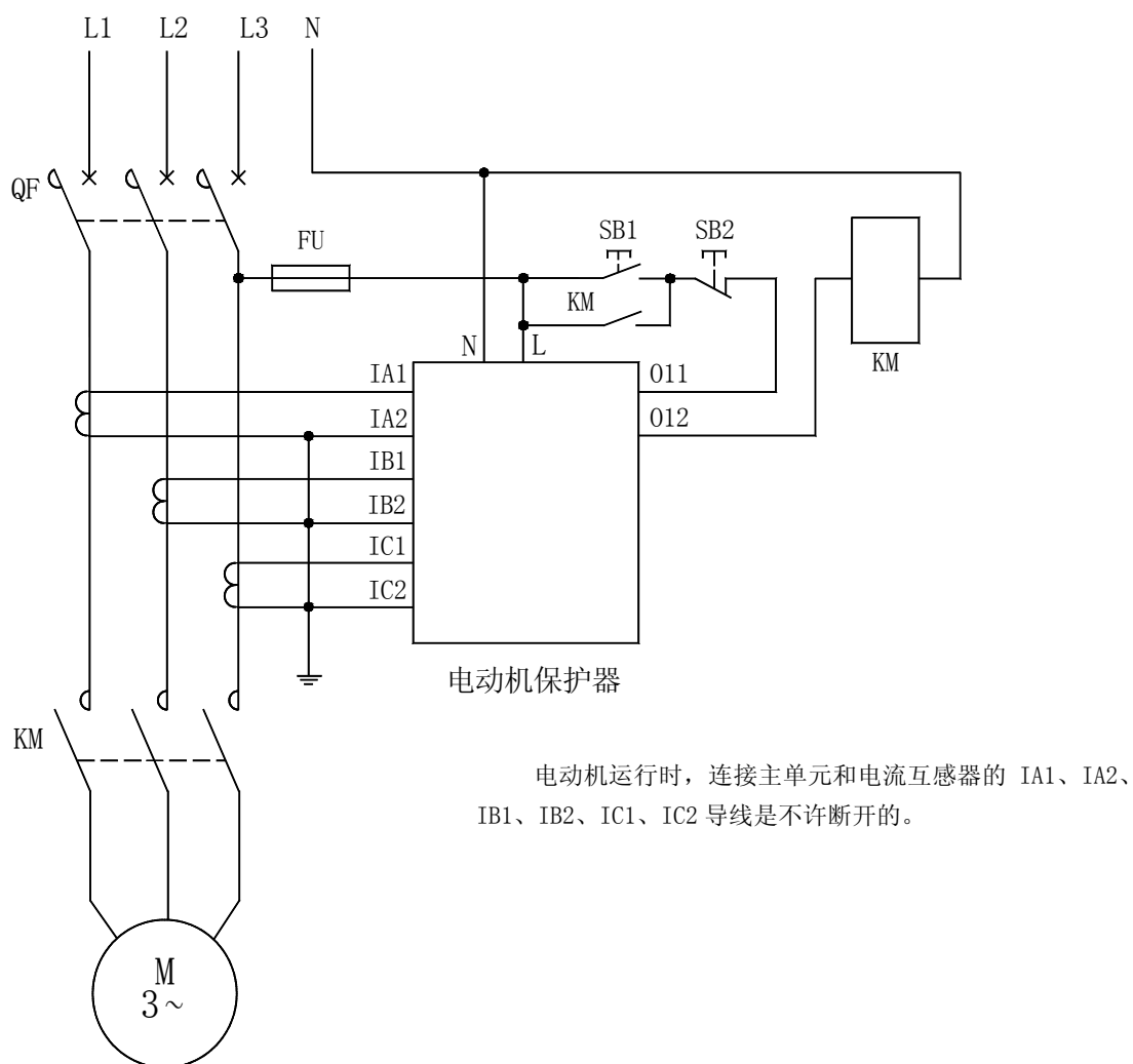
AMDG-X/E02□ 系列电动机保护器应用电气原理图
