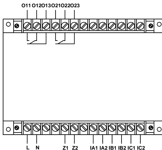
AMDG-X/E012 系列保护器主单元接线端子图
