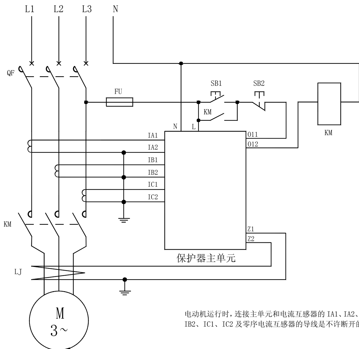
AMDG-X/E01□ 系列电动机保护器应用电气原理图
