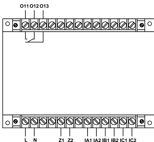
AMDG-X/E011 系列保护器主单元接线端子图
