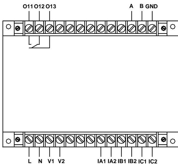
AMDG-□/241 系列保护器主单元接线端子图
