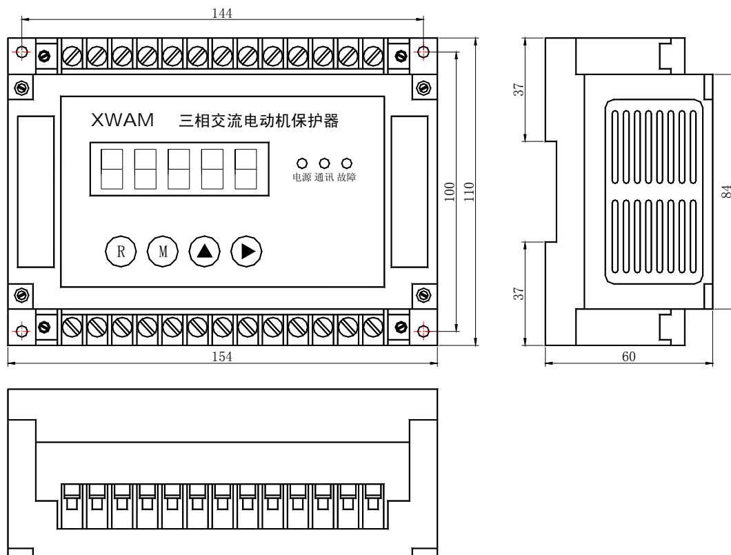
AMDG-□/24□ 系列电动机保护器主单元外形及安装孔尺寸
