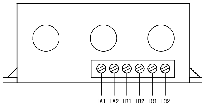
AMDG-□/24□ 系列保护器电流检测单元接线端子图
