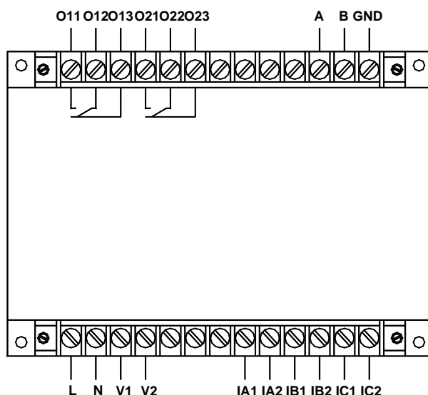
AMDG-□/242 系列保护器主单元接线端子图
