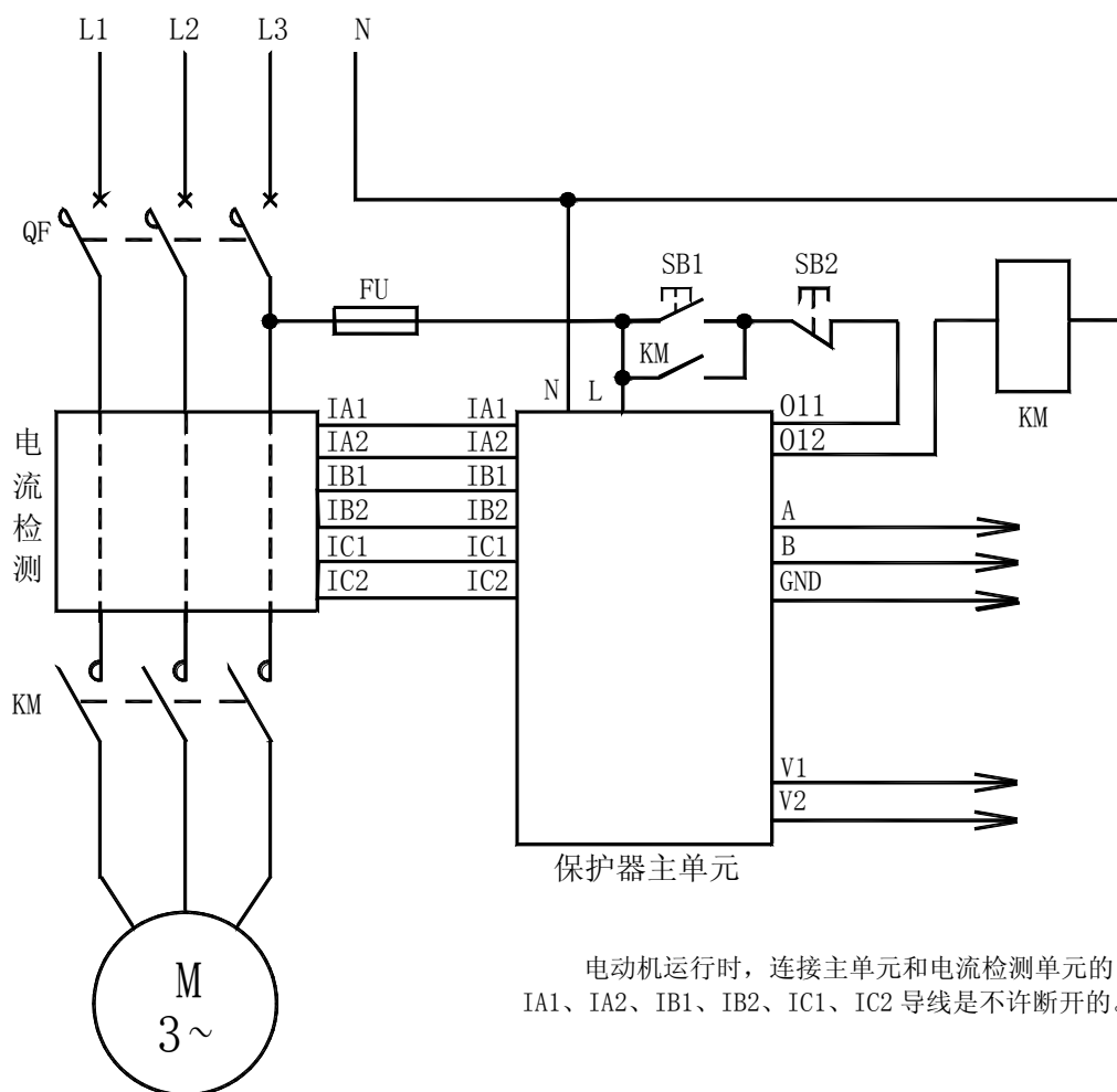
AMDG-□/□D24□ 系列电动机保护器应用电气原理
