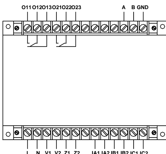
AMDG-□/ D212 系列保护器主单元接线端子图
