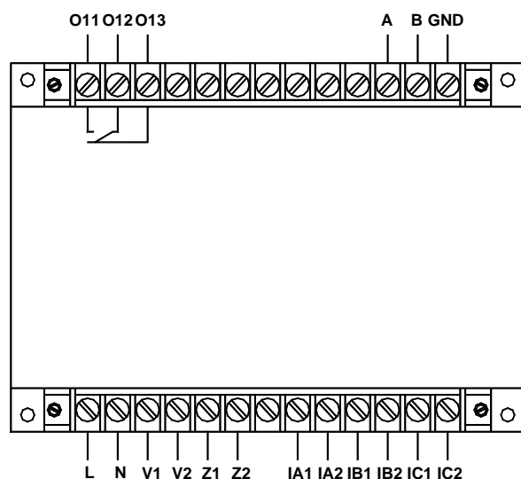
AMDG-□/ D211 系列保护器主单元接线端子图
