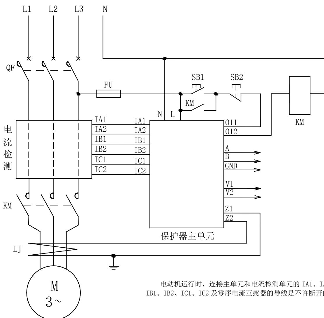
AMDG-□/ D21□ 系列电动机保护器应用电气原理图
