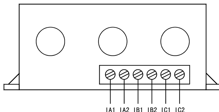
AMDG-□/ D21□ 系列保护器电流检测单元接线端子图
