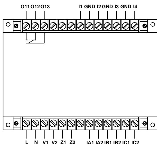
AMDG-□/□/171 系列保护器主单元接线端子图
