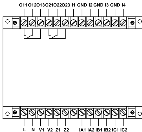
AMDG-□/□/172 系列保护器主单元接线端子图
