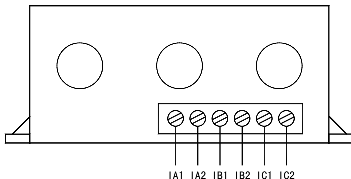
AMDG-□/□D17□ 系列保护器电流检测单元接线端子图
