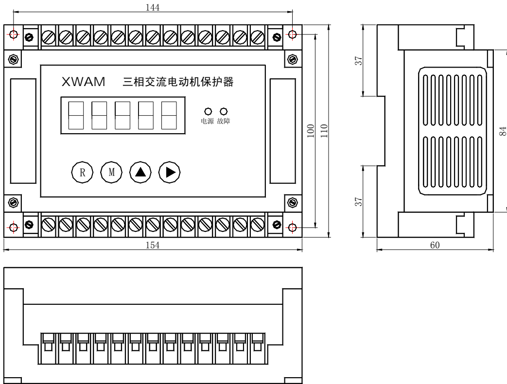
AMDG-□/ D17□ 系列电动机保护器主单元外形及安装孔尺寸
