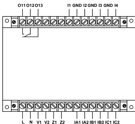
AMDG-□/ D161 系列保护器主单元接线端子图
