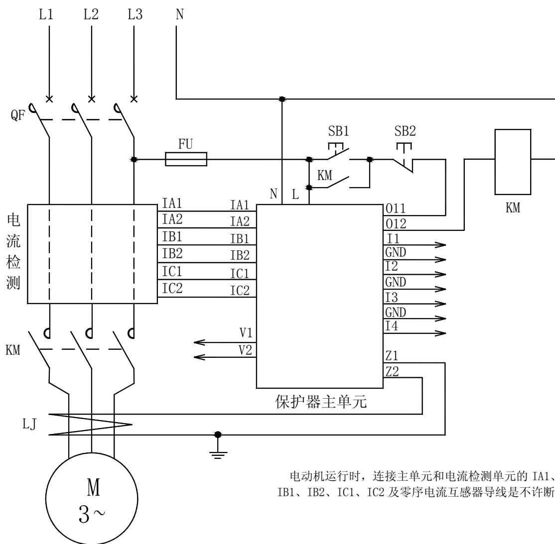
AMDG-□/□D16□ 系列电动机保护器应用电气原理图
