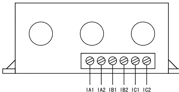
AMDG-□/ D16□ 系列保护器电流检测单元接线端子图
