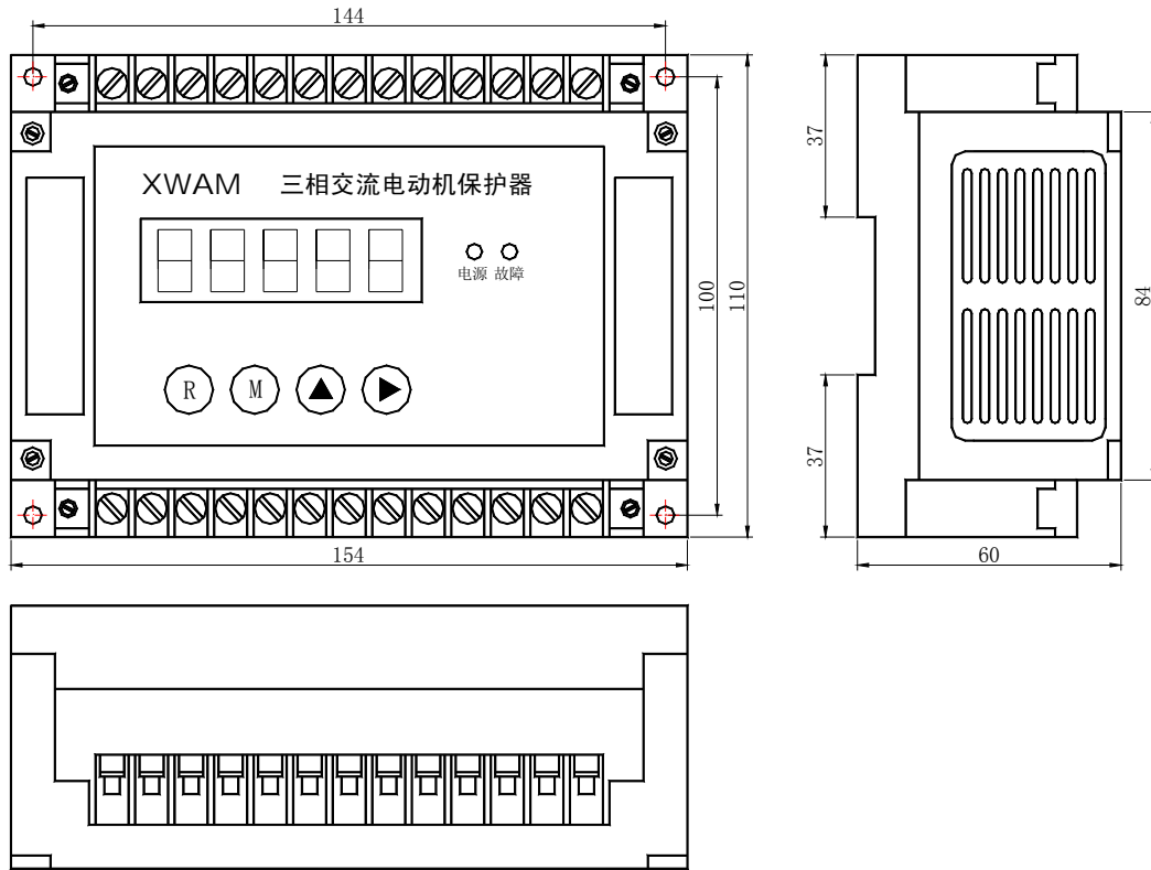
AMDG-□/□/16□ 系列电动机保护器主单元外形及安装孔尺寸
