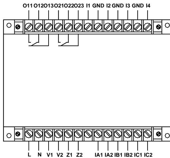
AMDG-□/ D162 系列保护器主单元接线端子图
