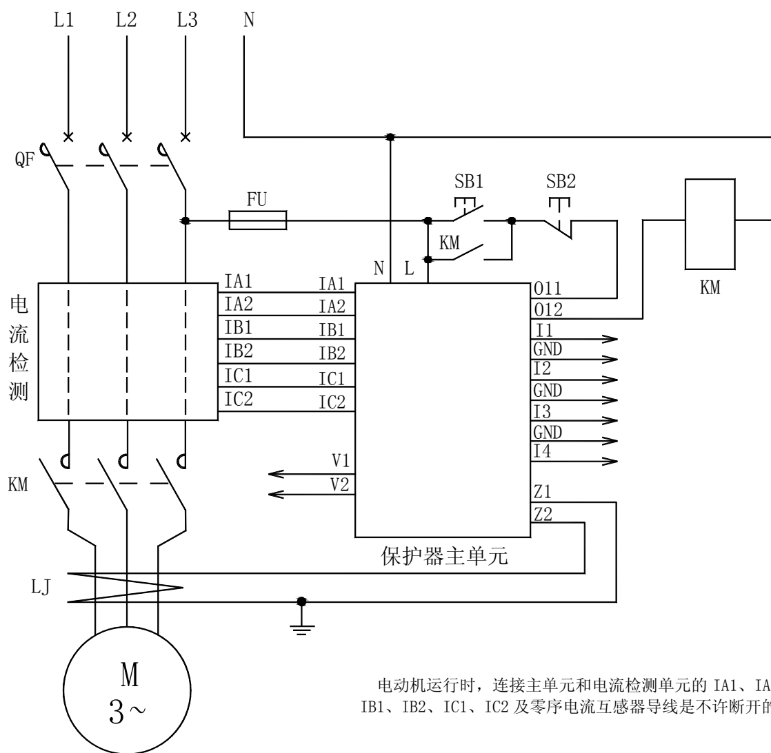
AMDG-□/□D11□ 系列电动机保护器应用电气原理图
