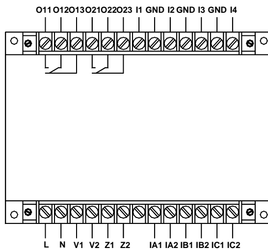
AMDG-□/ D112 系列保护器主单元接线端子图
