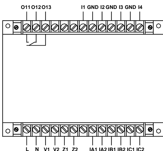
AMDG-□/ D111 系列保护器主单元接线端子图
