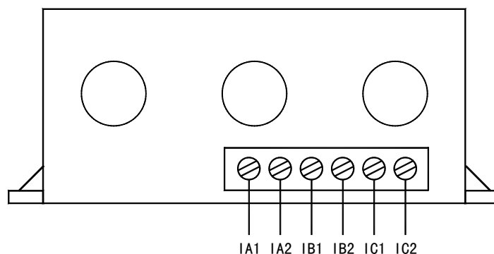
AMDG-□/ D11□ 系列保护器电流检测单元接线端子图
