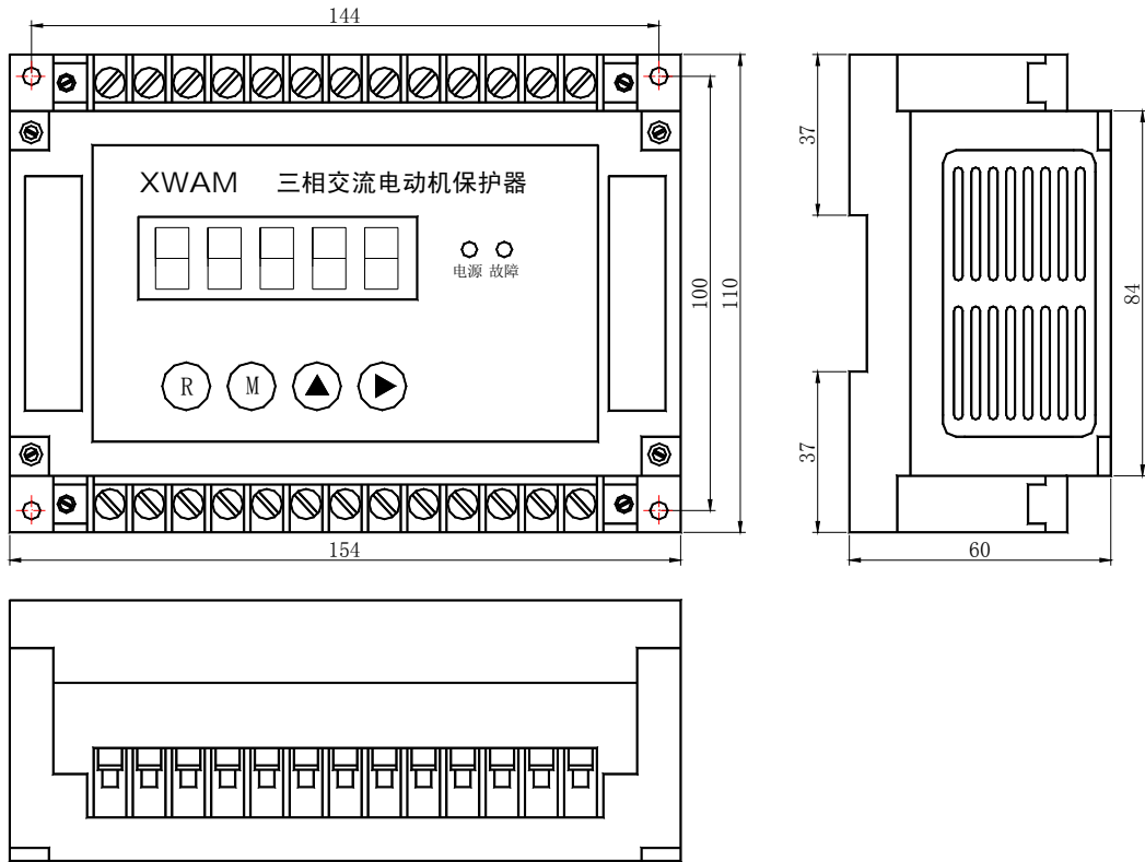
AMDG-□/ D11□ 系列电动机保护器主单元外形及安装孔尺寸
