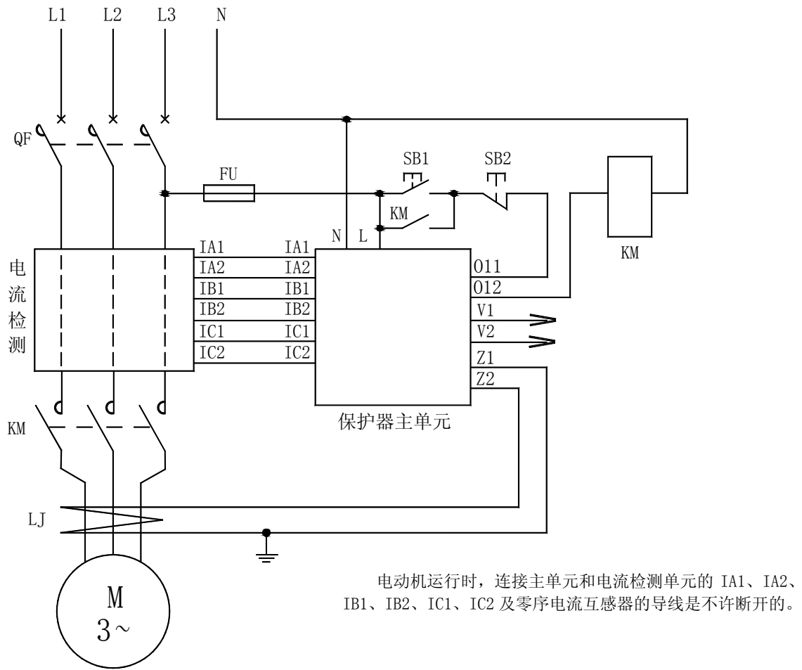
AMDG-□/DO7□ 系列电动机保护器应用电气原理图
