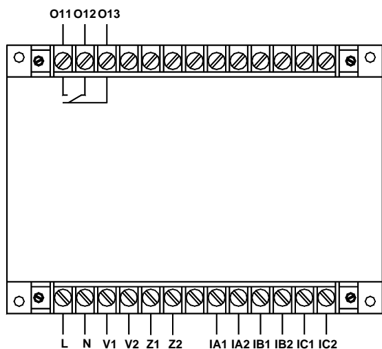
AMDG-□/DO71 系列保护器主单元接线端子图
