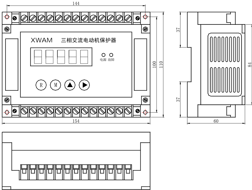
AMDG-□/DO7□ 系列电动机保护器主单元外形及安装孔尺寸
