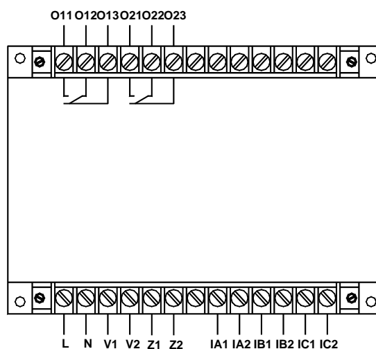
AMDG-□/DO72 系列保护器主单元接线端子图
