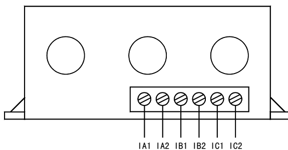
AMDG-□/DO7□ 系列保护器电流检测单元接线端子图
