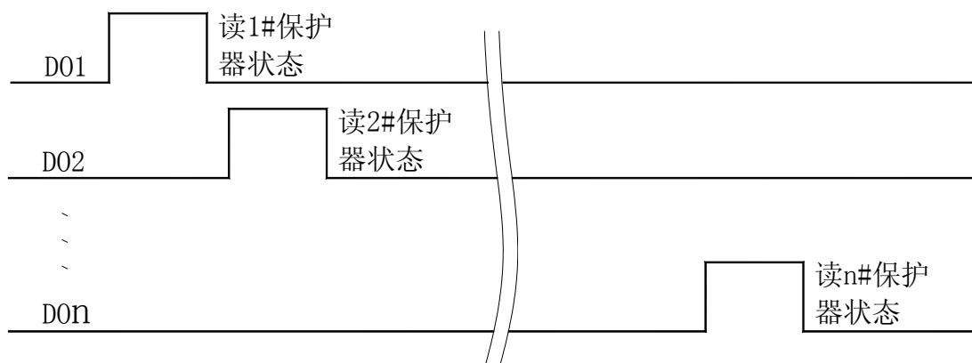
PLC 读取多台 AMDG-□/ C611 系列电动机保护器时序图
