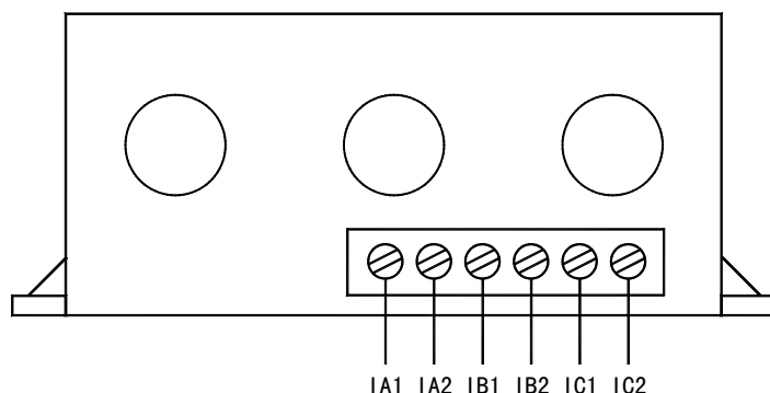
AMDG-□/□C611 系列保护器电流检测单元接线端子图
