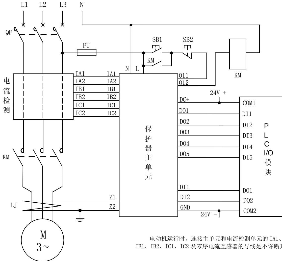
AMDG-□/C611 系列电动机保护器 DO 连接 PLC 电气原理图
