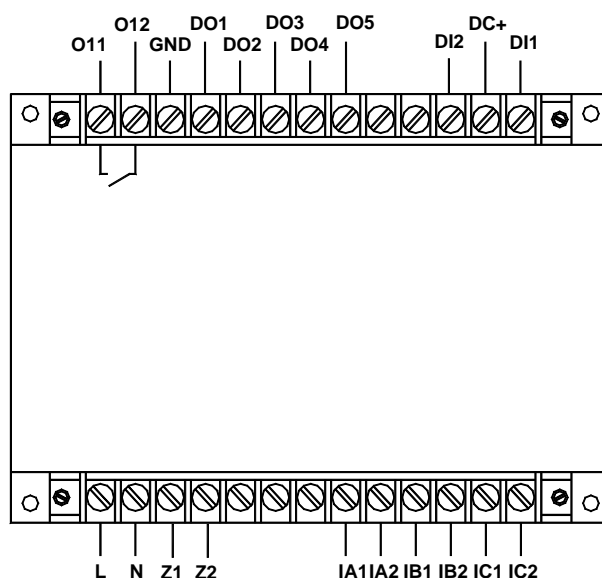
AMDG-□/611 系列保护器主单元接线端子图
