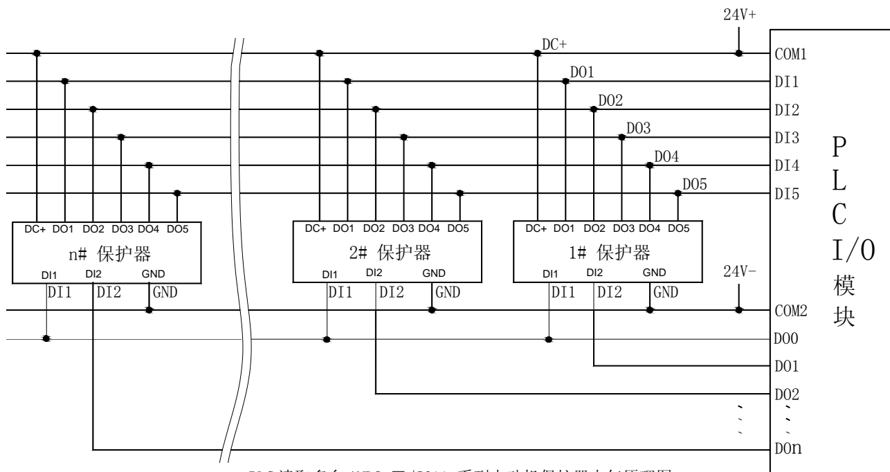
PLC 读取多台 AMDG-□/ C611 系列电动机保护器电气原理图
