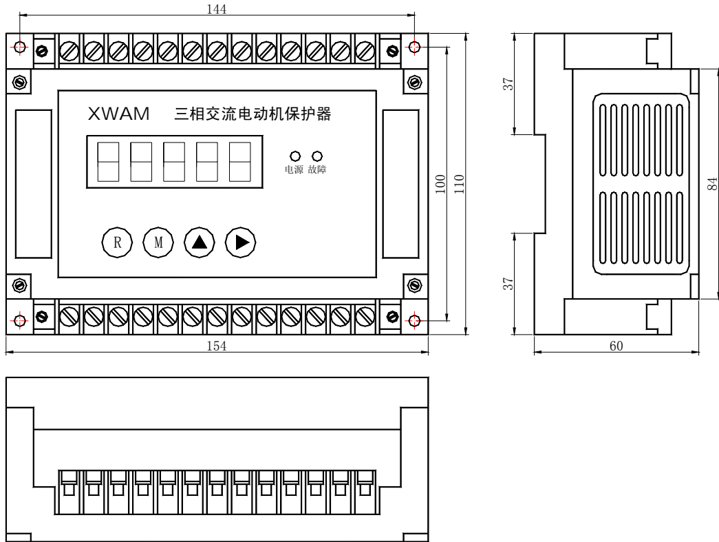
AMDG-□/ C611 系列电动机保护器主单元外形及安装孔尺寸
