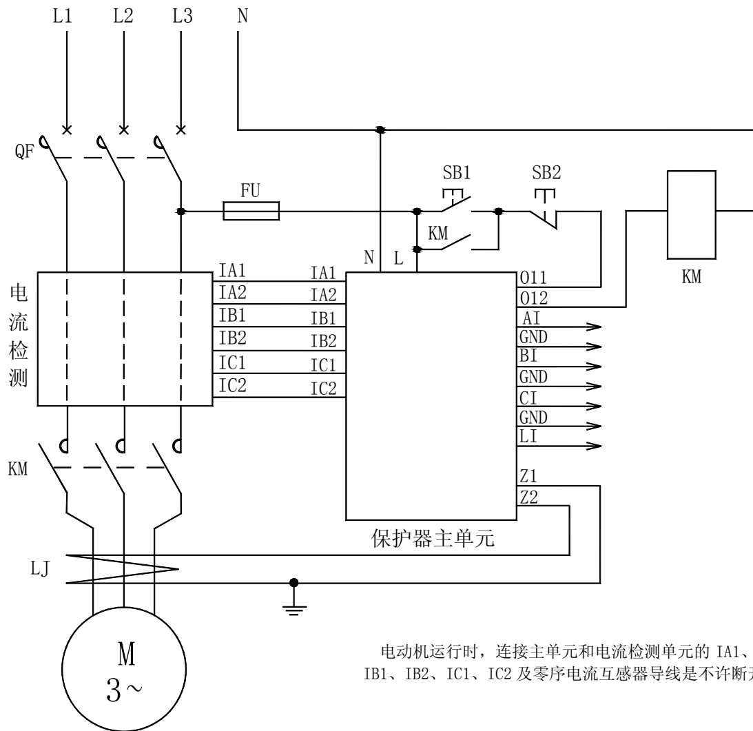
AMDG-□/□C15□ 系列电动机保护器应用电气原理图
