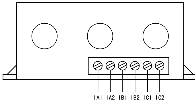
AMDG-□/□/15□ 系列保护器电流检测单元接线端子图
