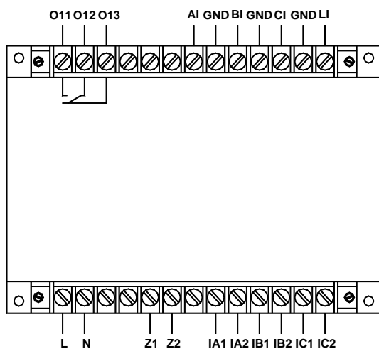
AMDG-□/□/151 系列保护器主单元接线端子图
