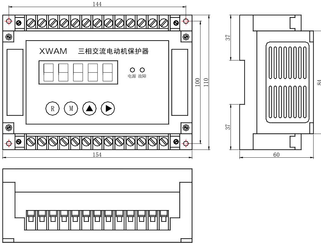
AMDG-□/□/15□ 系列电动机保护器主单元外形及安装孔尺寸
