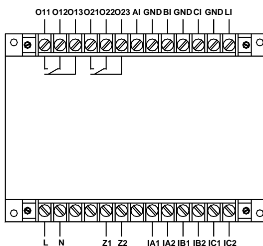
AMDG-□/□/152 系列保护器主单元接线端子图
