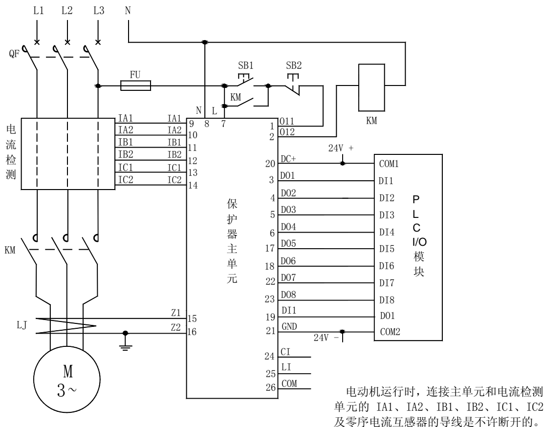
AMDP-□/C711 系列电动机保护器 D0 连接 PLC 电气原理图
