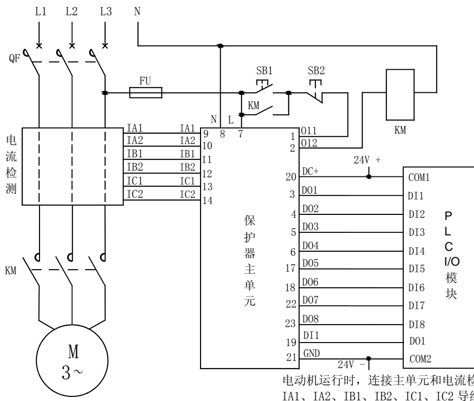
AMDP-□/C501、AMDP-□/C521 系列电动机保护器 DO 连接 PLC 电气原理图
