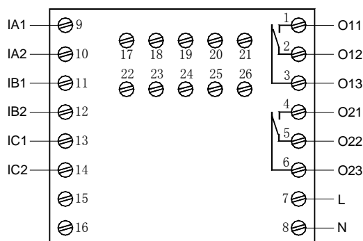
AMDP-□/C002、AMDP-□/C022 主单元端子图
