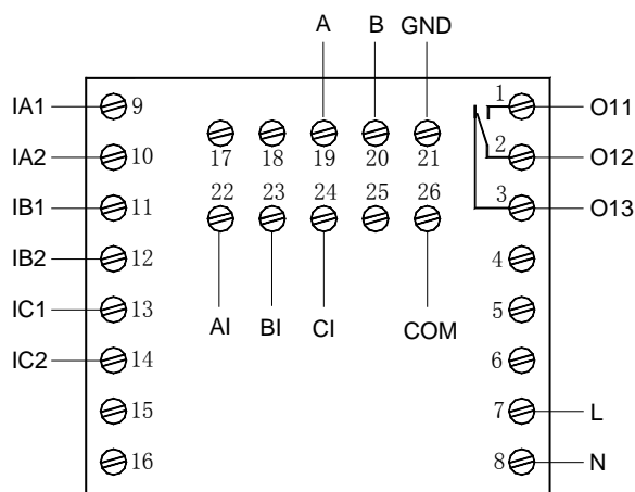
AMDP-□/C401、AMDP-□/C421 主单元接线端子图
