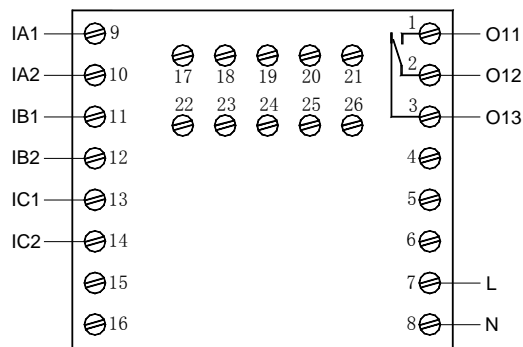
AMDP-□/C001、AMDP-□/C021 主单元端子图
