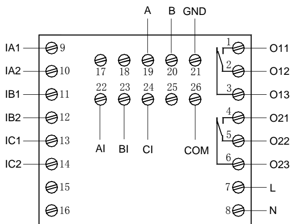
AMDP-□/C402、AMDP-□/C422 主单元接线端子图
