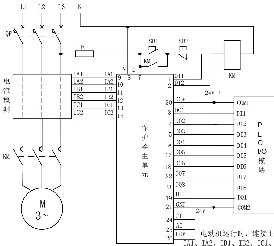
AMDP-□/C701、AMDP-□/C721 保护器 D0 连接 PLC 电气原理图
