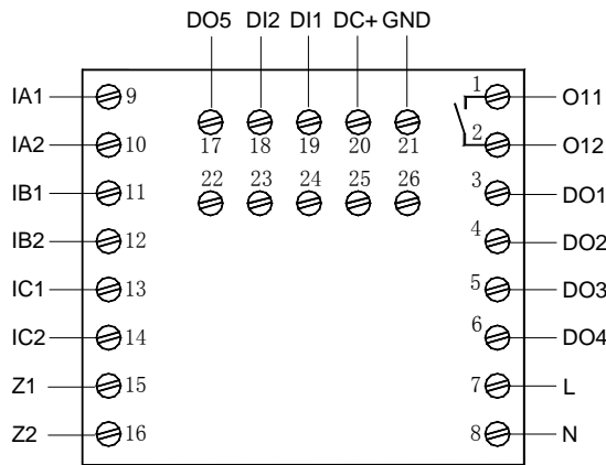
AMDP-□/C611 系列保护器主单元接线端子图
