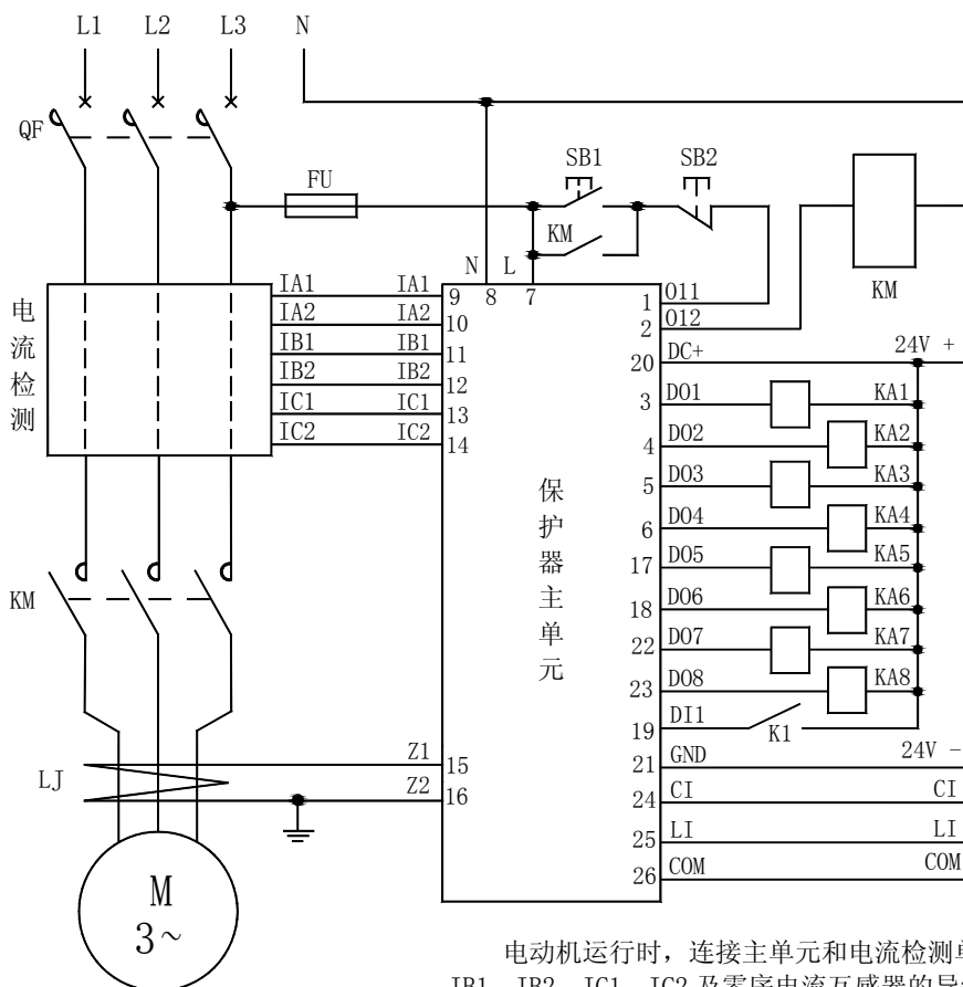
AMDP-□/C711 系列电动机保护器 DO 连接继电器电气原理图
