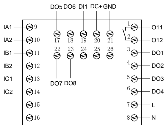
AMDP-□/C501、AMDP-□/C521 主单元接线端子图
