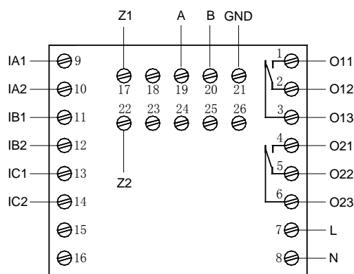
AMDP-□/C212、AMDP-□/C312 主单元端子图
