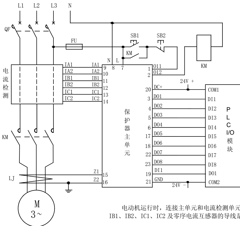
AMDP-□/C511 系列电动机保护器 D0 连接 PLC 电气原理图
