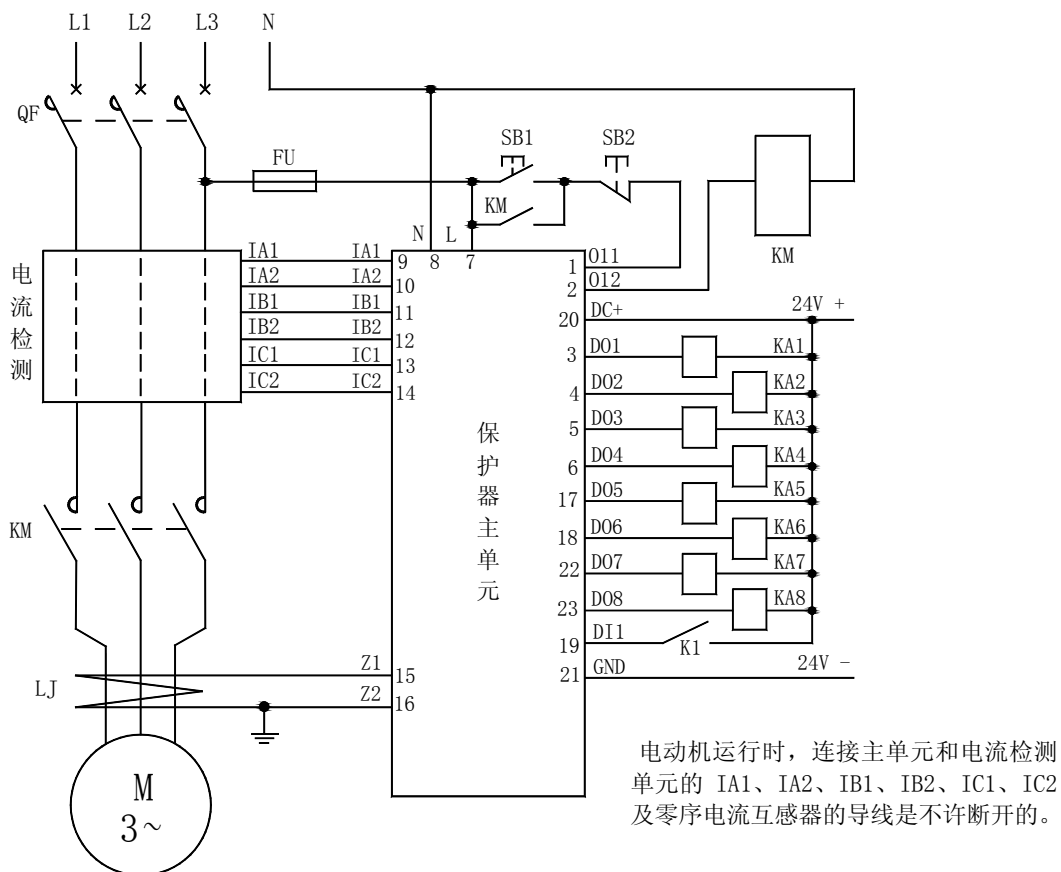
AMDP-□/C511 系列电动机保护器 DO 连接继电器电气原理图
