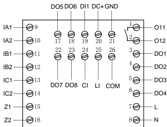
AMDP-□/C711 系列保护器主单元接线端子图
