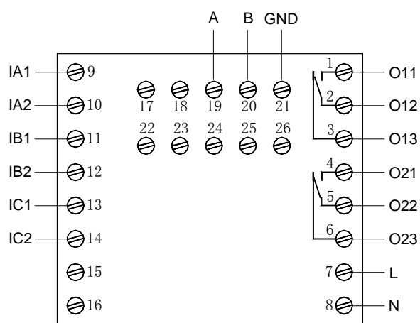
AMDP-□/C202、AMDP-□/C222 主单元端子图
