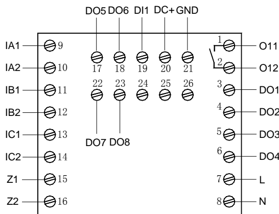
AMDP-□/C511 系列保护器主单元接线端子图
