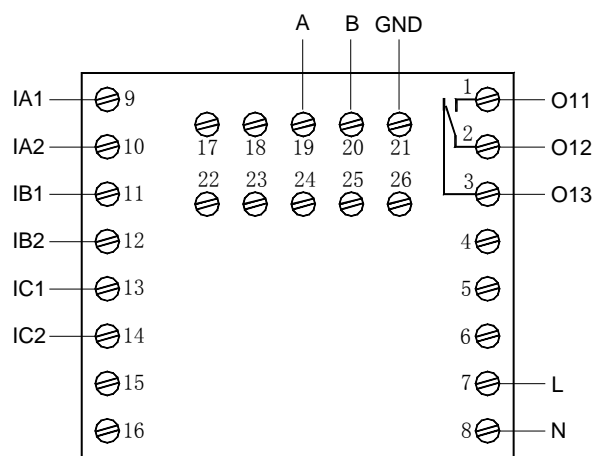
AMDP-□/C201、AMDP-□/C221 主单元端子图
