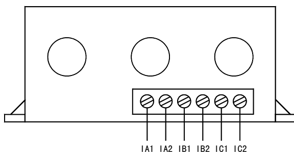
AMDP-□/C 系列电动机保护器电流检测单元接线端子图
