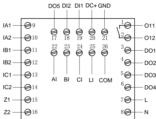
AMDP-□/C811 系列保护器主单元接线端子图
