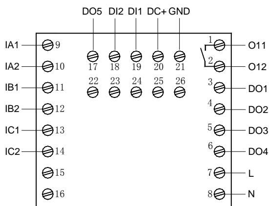
AMDP-□/C601、AMDP-□/C621 主单元接线端子图
