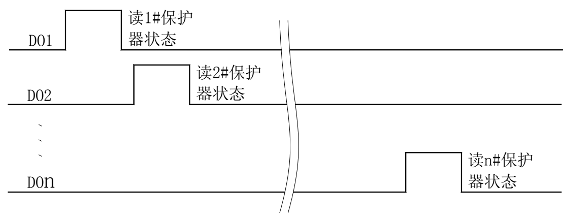
PLC 读取多台 AMDP-□/C6、AMDP-□/C8 系列电动机保护器时序图
