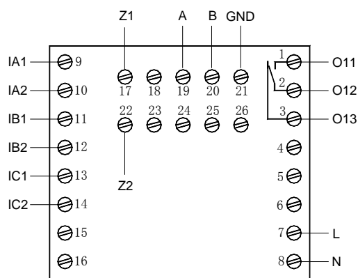
AMDP-□/C211、AMDP-□/C311 主单元端子图
