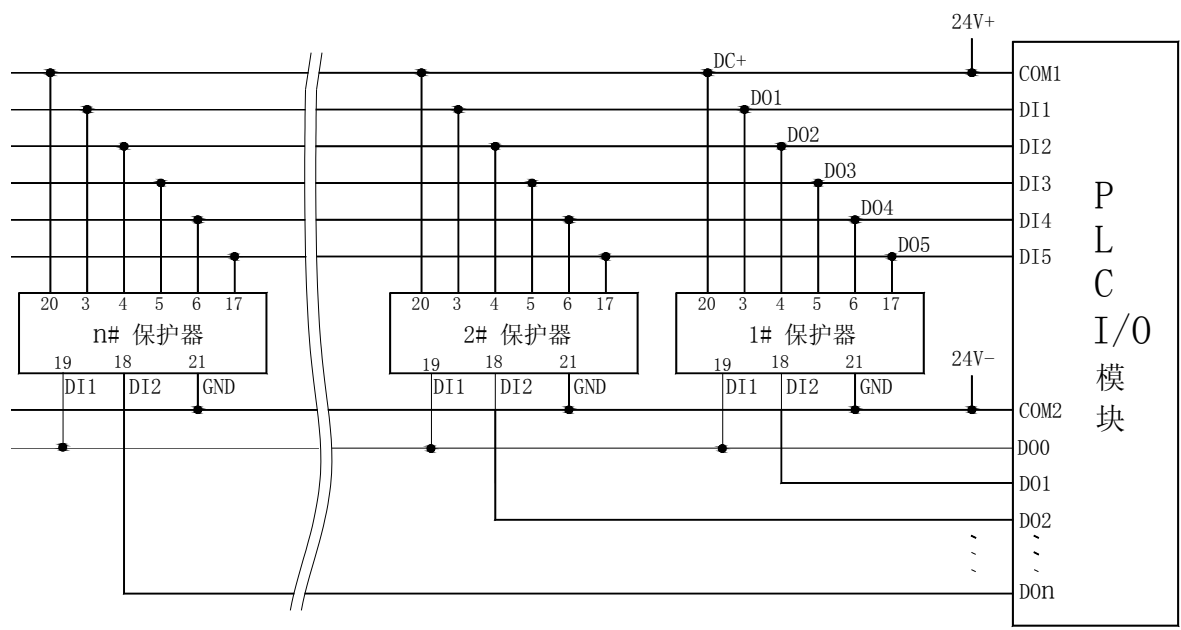
PLC 读取多台 AMDP-□/C6、AMDP-□/C8 系列电动机保护器电气原理图
