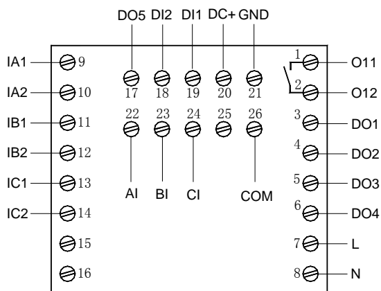
AMDP-□/C801、AMDP-□/C821 主单元接线端子图
