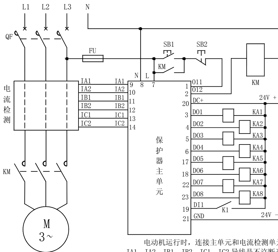
AMDP-□/C501、AMDP-□/C521 系列电动机保护器 DO 连接继电器电气原理图
