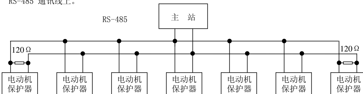
图 6 电动机保护器 RS-485 通讯网络连接图
